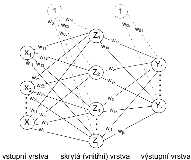
Obrázek 3.3: Příklad neuronové sítě (volně převzato z (VolnÁ, 2008))
